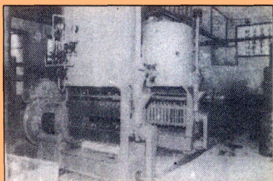
200 型榨油机
