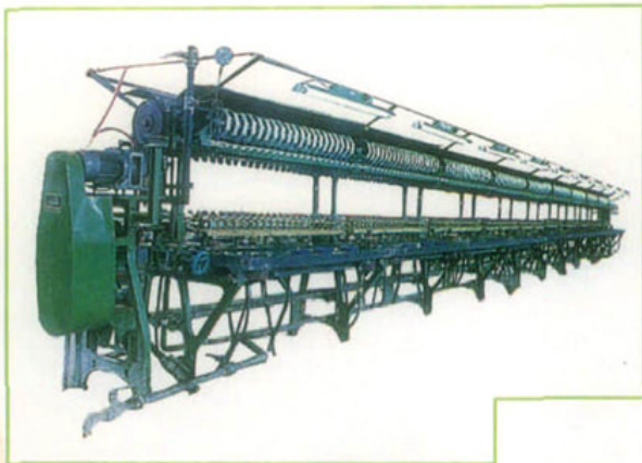
CD801A立缫机 (四川省纺织机械厂生产)
