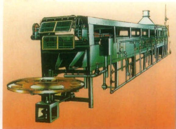
FD301型煮茧机 (成都纺织机械厂生产)
